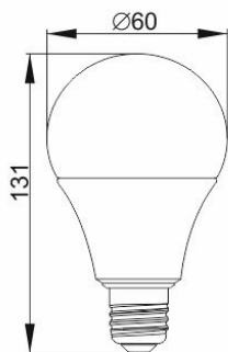
Рисунок 2 – Лампа LED-A60, 13 Вт, 15 Вт, 20 Вт цоколь E27
