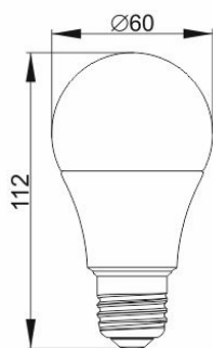
Рисунок 1 – Лампа LED-A60, 7 Вт, цоколь E27
