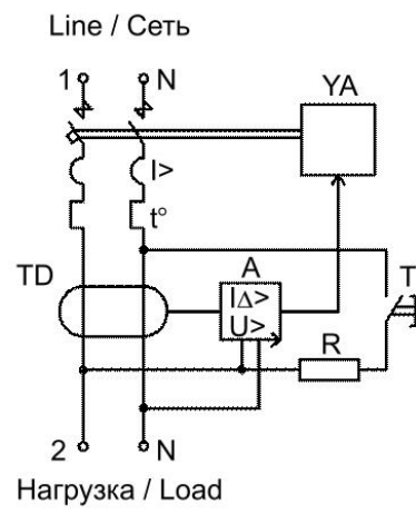
Рисунок 1. Схема электрическая принципиальная
