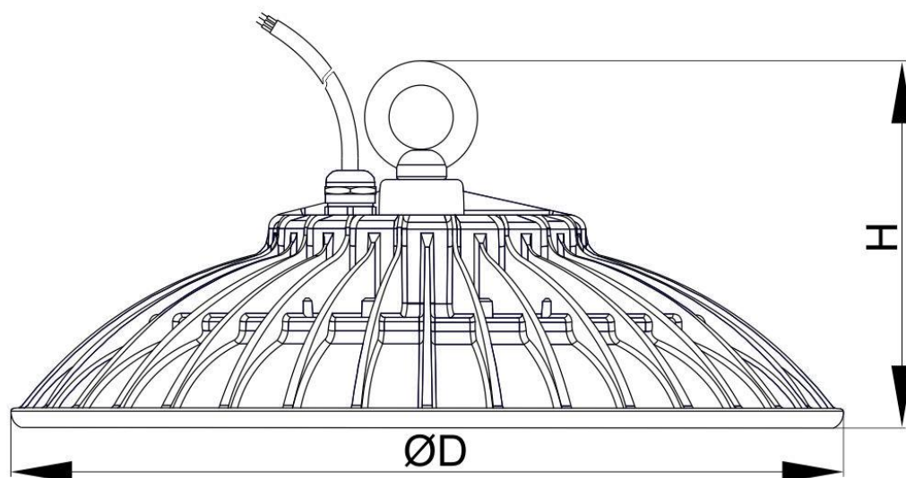
Рисунок 1. Габаритные размеры светильников ДСП 3004-3019 PRO
