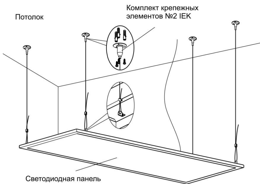
Рисунок 2. Подвесной монтаж светодиодной панели
