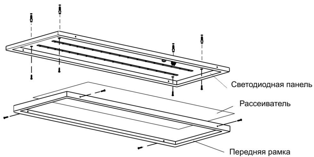
Рисунок 1. Накладной монтаж светодиодной панели
