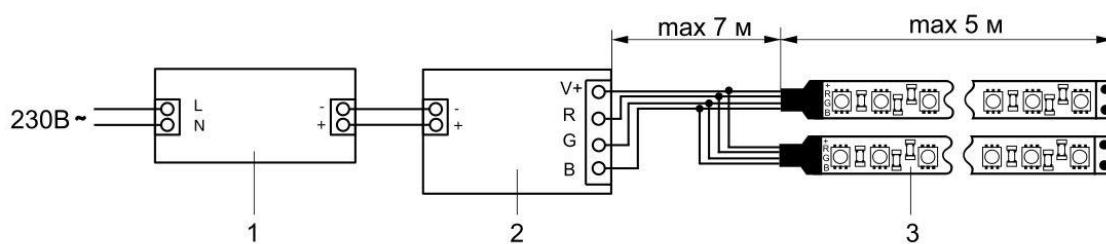
Рисунок 2 – Схема подключения RGB светодиодной ленты к блоку питания и контроллеру
