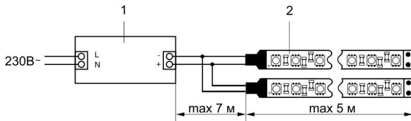
Рисунок 1 – Схема подключения одноцветной светодиодной ленты
