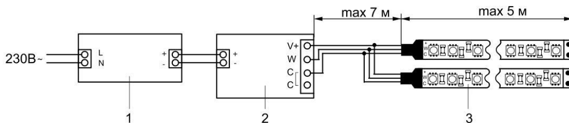
Рисунок 3 – Схема подключения мультисветодиодной ленты к блоку питания и контроллеру
