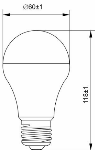
Рисунок 1. Габаритный чертеж - Лампа светодиодная IT-L220E27-YR004-WB
