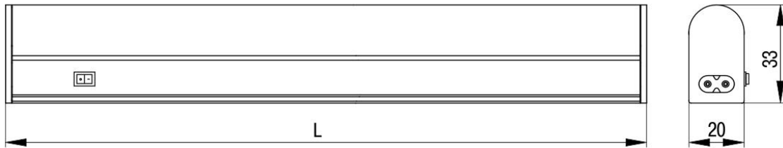
Рисунок 1 - Габаритные размеры светильников
