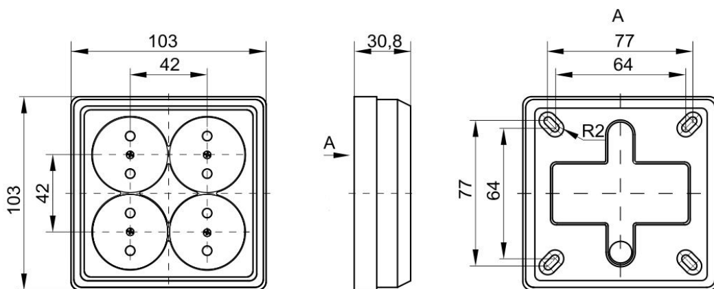
Рисунок 7. Розетки PC24-2-ОБ; PC24-2-ОК; PC24-2-ОС; PC24-2-ОД.
