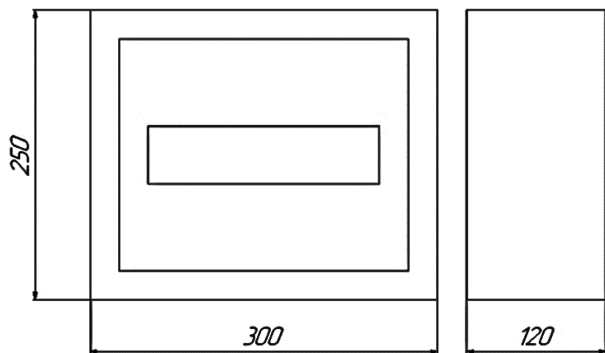
Рисунок 1. Габаритные и установочные размеры щитков осветительных ОЦВ-6
