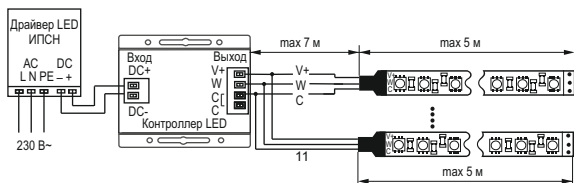
Рисунок 7 – Схема параллельного подключения мультислойной светодиодной ленты к блоку питания и контроллеру
