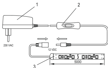
Рисунок 13 – Подключение LSR1-1-060-20-1-2XD12-S3
