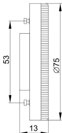
Рисунок 1 – Лампа LED-T75, 4 Вт, 6 Вт, 8 Вт, цоколь GX53
