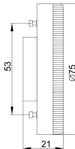
Рисунок 2 – Лампа LED-T75, 10 Вт, цоколь GX53
