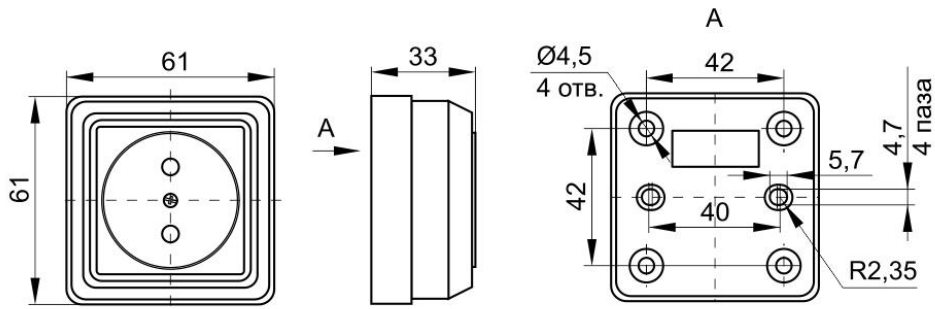
Рисунок 1. Розетки РС20-2-ОБ; РС20-2-ОКм; РС20-2-ОС; РС20-2-ОД; РСш20-2-ОБ; РСш20-2-ОКм; РСш20-2-ОС; РСш20-2-ОД.
