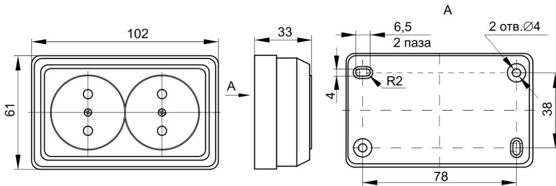
Рисунок 3. Розетки РС22-2-ОБ; РС22-2-ОКм; РС22-2-ОС; РС22-2-ОД; РСш22-2-ОБ; РСш22-2-ОКм; РСш22-2-ОС; РСш22-2-ОД.
