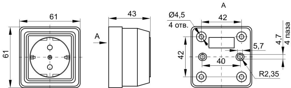
Рисунок 2. Розетки РС20-3-ОБ; РС20-3-ОКм; РС20-3-ОС; РС20-3-ОД; РСш20-3-ОБ; РСш20-3-ОКм; РСш20-3-ОС; РСш20-3-ОД.
