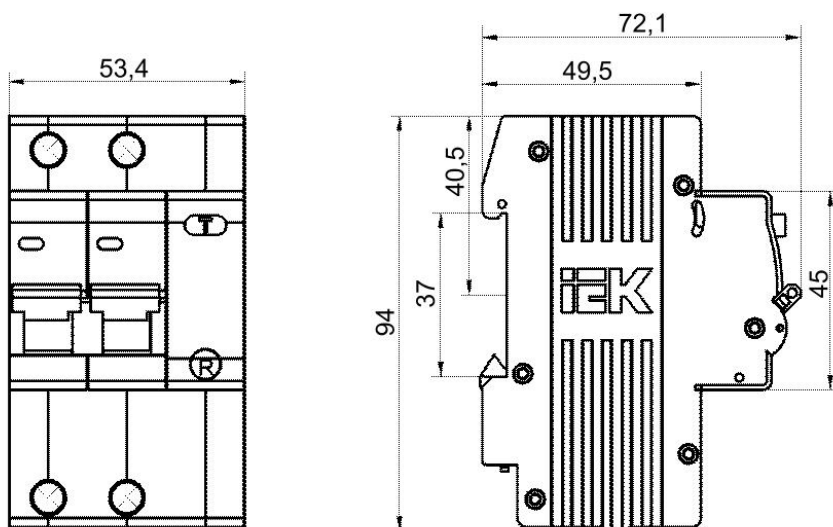
Рисунок 1. Габаритные размеры АД12
