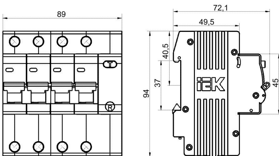
Рисунок 2. Габаритные размеры АД14
