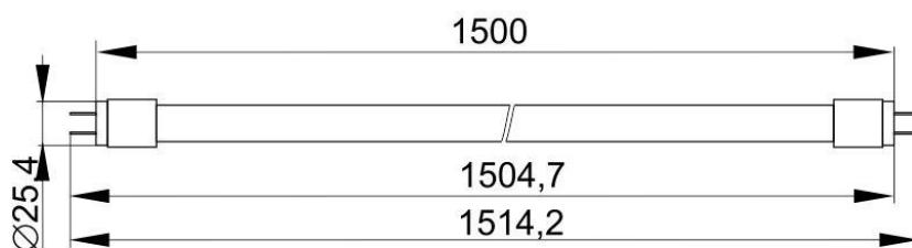
Рисунок 3 – Лампа LED-T8, 24 Вт, цоколь G13
