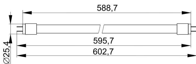
Рисунок 1 – Лампа LED-T8, 10 Вт, 13 Вт, цоколь G13
