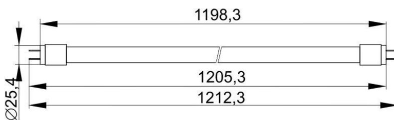
Рисунок 2 – Лампа LED-T8, 18 Вт, 20 Вт, 25 Вт, 30 Вт, 40 Вт, цоколь G13
