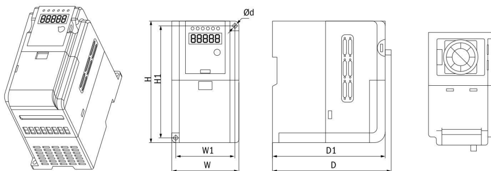
Рисунок 1. Габаритные размеры векторных преобразователей частоты серии A150 (Габарит 1)
