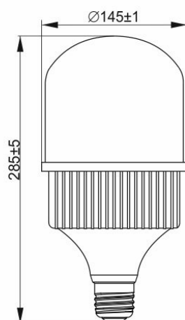
Рисунок 5 – Лампа LED- HP, 120 Вт, цоколь E40
