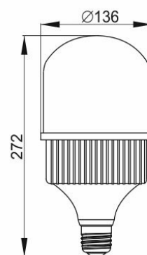
Рисунок 4 – Лампа LED-HP, 80 Вт, 100 Вт, цоколь E40
