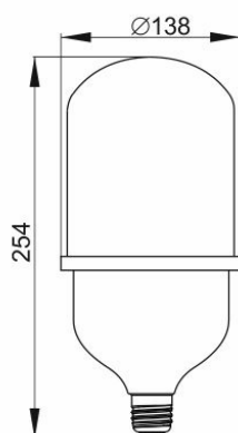
Рисунок 2 – Лампа LED-HP, 50 Вт, цоколь E40
