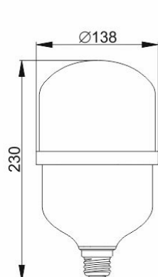
Рисунок 1 – Лампа LED-HP, 50 Вт, цоколь E27
