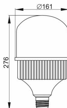
Рисунок 3 – Лампа LED-HP, 65 Вт, цоколь E40
