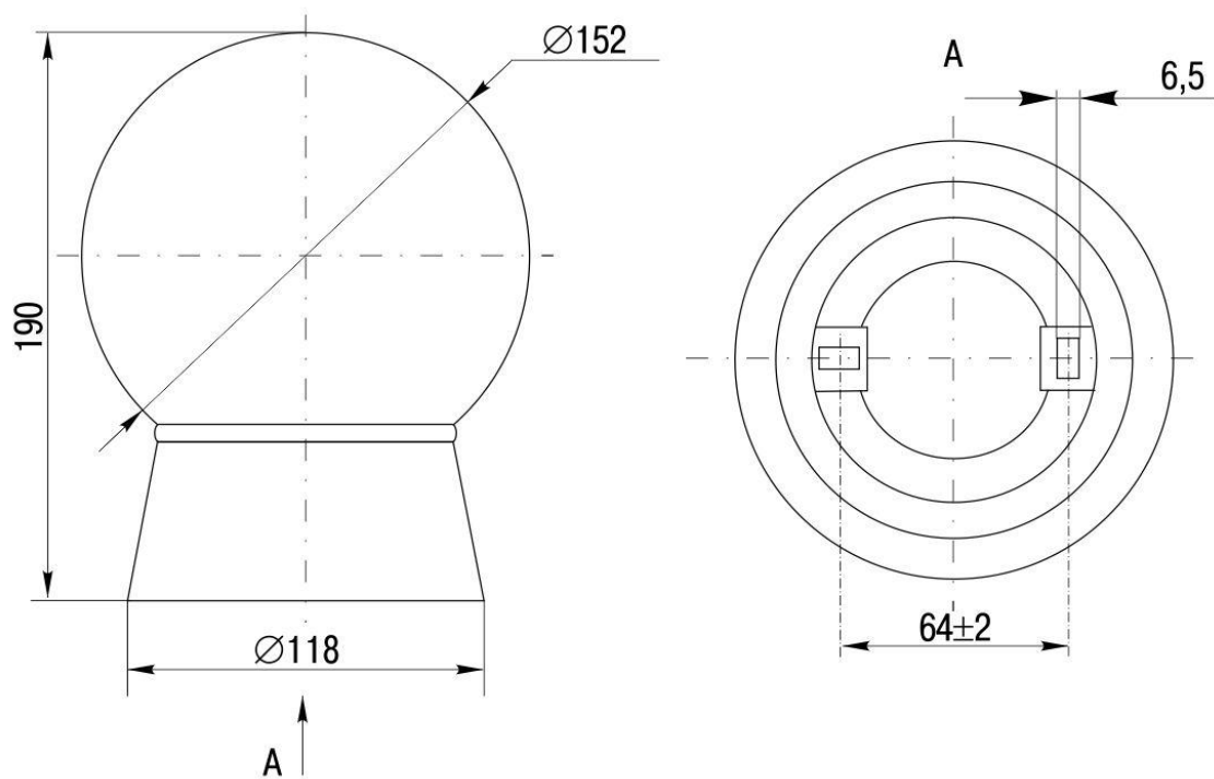
Рисунок 1 – Габаритные и установочные размеры светильника НПП 9101
