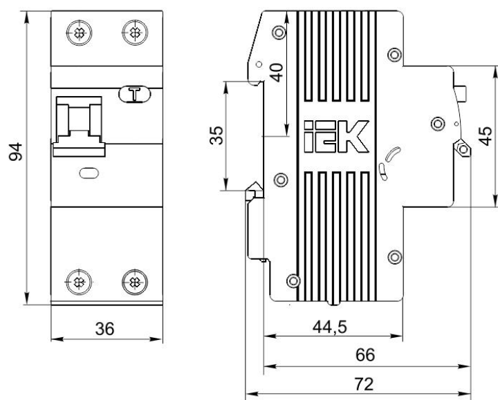
Рисунок 2 – Габаритные размеры АВДТ32 (In 50 А, 63 А)
