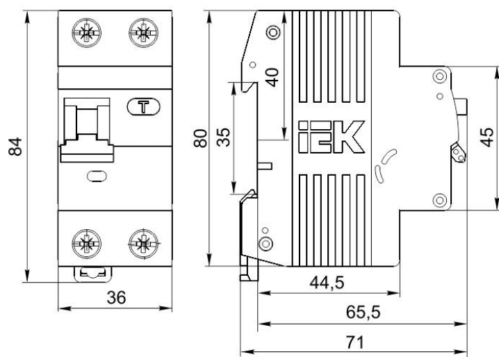
Рисунок 1 – Габаритные размеры АВДТ32 (In 6-40 А)
