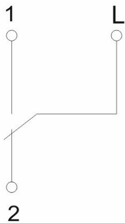
Рисунок 1 – Электрическая схема выключателя ВС10-1-6-БрХ*
