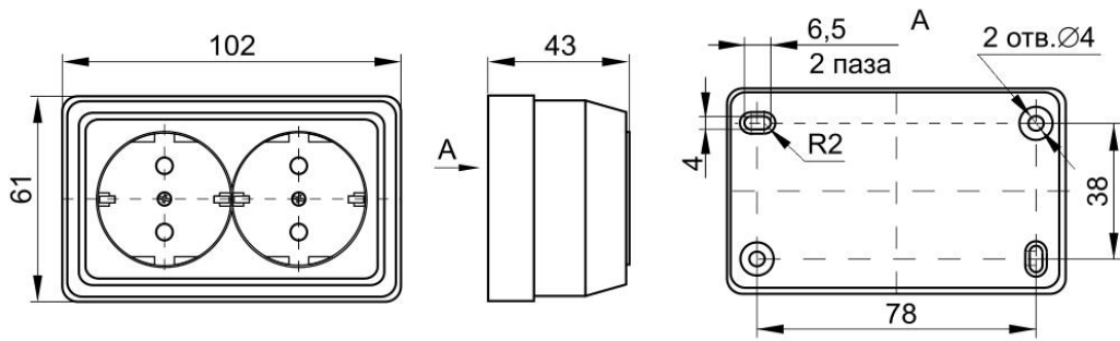
Рисунок 4. Розетки РС22-3-ОБ; РС22-3-ОКм; РС20-3-ОС; РС20-3-ОД; РСш20-3-ОБ; РСш20-3-ОКм; РСш20-3-ОС; РСш20-3-ОД.
