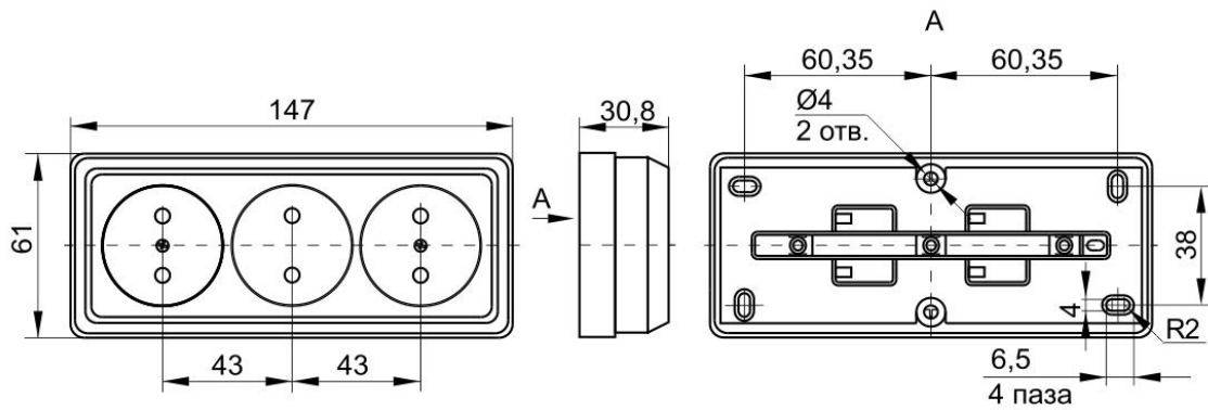
Рисунок 5. Розетки РС23-2-ОБ; РС23-2-ОК; РС23-2-ОС; РС23-2-ОД.
