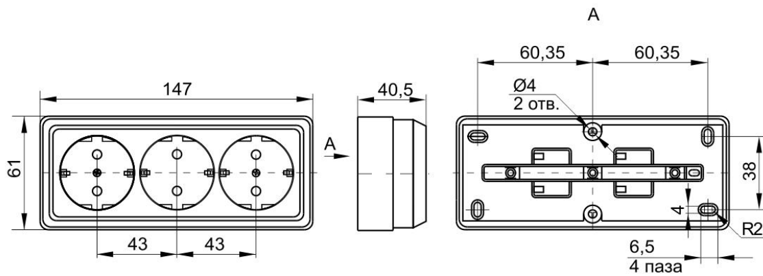
Рисунок 6. Розетки РС23-3-ОБ; РС23-3-ОК; РС23-3-ОС; РС23-3-ОД.
