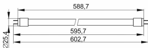
Рисунок 1– Лампа LED–Т8, 10 Вт, 13 Вт, цоколь G13
