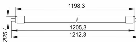
Рисунок 2– Лампа LED–Т8, 18 Вт, 20 Вт, 25 Вт, 30 Вт, 40 Вт, цоколь G13
