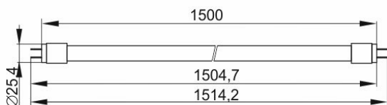
Рисунок 3– Лампа LED–Т8, 24 Вт, цоколь G13
