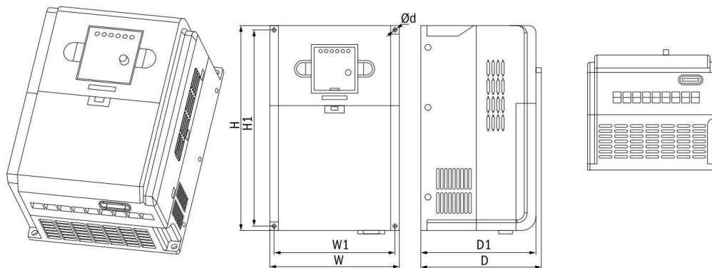
Рисунок 1. Габаритные размеры векторных преобразователей частоты серии A150 (Габарит 4)
