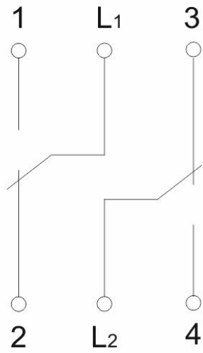
Рисунок 1 – Электрическая схема выключателя ВВС10-2-6-БрХ*
