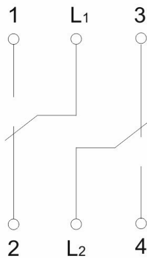
Рисунок 1 – Электрическая схема выключателя BBC10-2-6-BrX*
