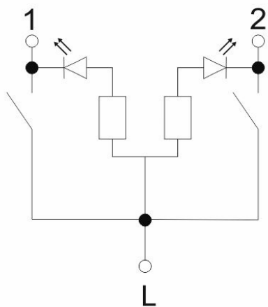
Рисунок 1 – Электрическая схема выключателя VC10-2-1-BrX*
