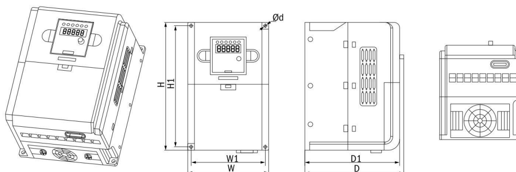
Рисунок 1. Габаритные размеры векторных преобразователей частоты серии A150 (Габарит 3)
