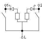
h) выключатель двухклавишный с индикацией / 2-gang switch with indication / индикациясы бар екі пернелі ажыратқыш / intrerupator dublu cu indicatie / хоёр даралттай led гэрэлтэй унтраалга / indikatsiyali ikkita klavishli o'chirgich
