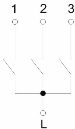
Рисунок 1 – Электрическая схема выключателя ВС10-3-0-БрХ*
