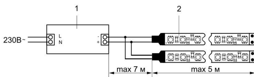
Рисунок 1 – Схема подключения монохромной и цветной светодиодной ленты к блоку питания
