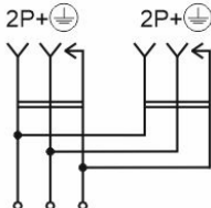
д) двухместная с заземлением
