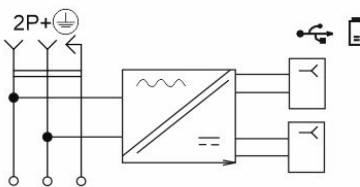
е) розетка с USB- разъемами
