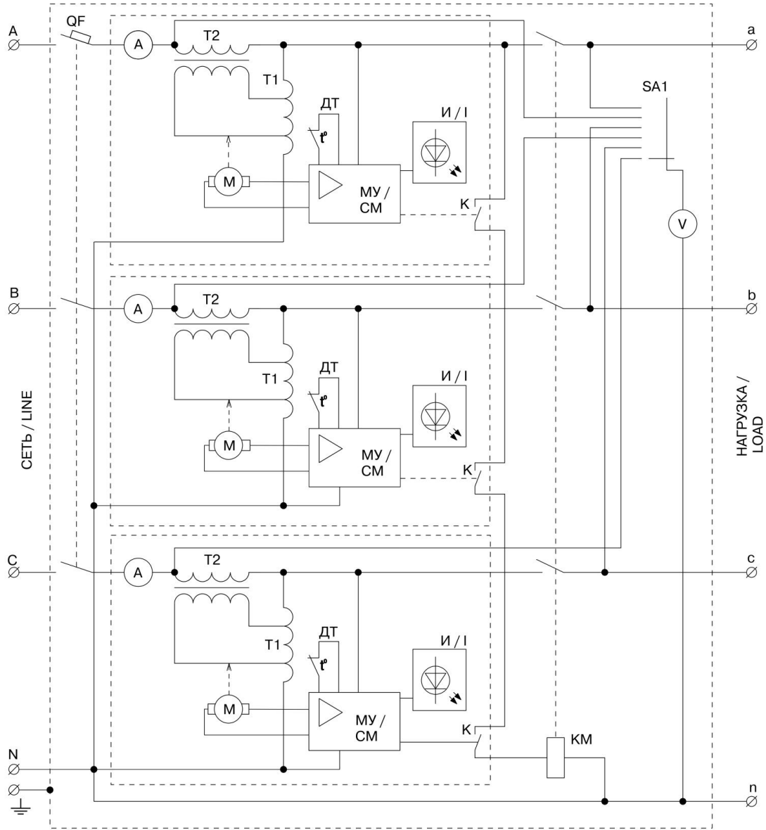
Рисунок 16 – Структурные схемы стабилизаторов: СНИЗ-15 кВА; СНИЗ-20 кВА; СНИЗ-30 кВА; СНИЗ-45 кВА; СНИЗ-60 кВА с дополнительным вольтодобавочным трансформатором
