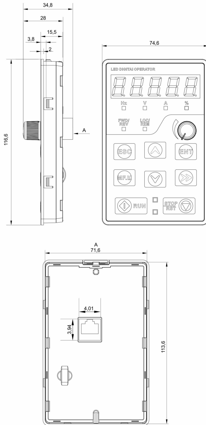
Рисунок 1. Габаритные размеры клавиатуры 3,7÷450 кВт
