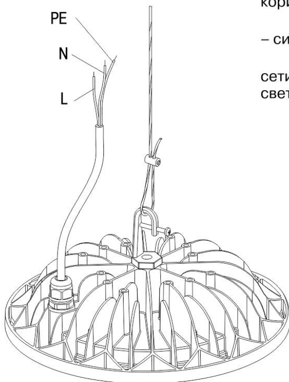
Рисунок 1 - Монтаж и подключение светильников
