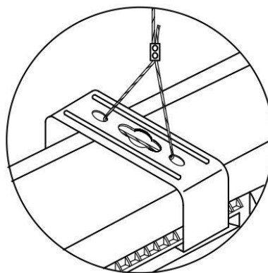
Рисунок 3. Монтаж светильника на подвесах
