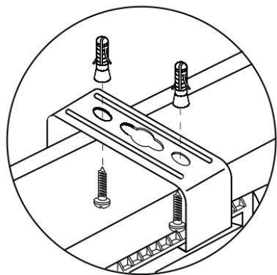
Рисунок 2. Монтаж светильника на рабочую поверхность
