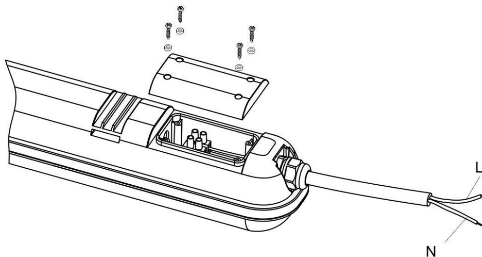
Рисунок 1. Подключение светильника
