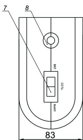
Рисунок 2. Левая боковая панель стабилизатора
