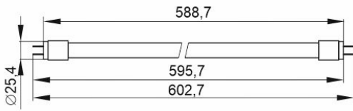
Лампа LED-T8, 10 Вт, 13 Вт цоколь G13
