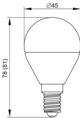
Лампа LED-G45, 3 Вт, 5 Вт цоколь E14
