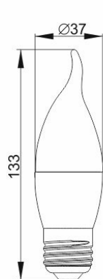
Рисунок 6 – Лампа LED-CB35, 5 Вт, 7 Вт, цоколь E27
