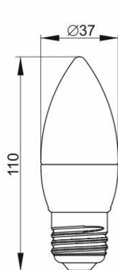
Рисунок 4 – Лампа LED-C35, 7 Вт, 9 Вт, цоколь E27
