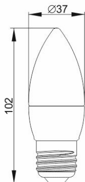
Рисунок 2 – Лампа LED-C35, 5 Вт, цоколь E27
