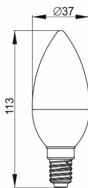
Рисунок 3 – Лампа LED-C35, 7 Вт, 9 Вт, цоколь E14
