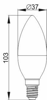
Рисунок 1 – Лампа LED-C35, 5 Вт, цоколь E14
