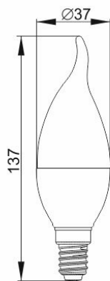
Рисунок 5 – Лампа LED-CB35, 5 Вт, 7 Вт, цоколь E14
