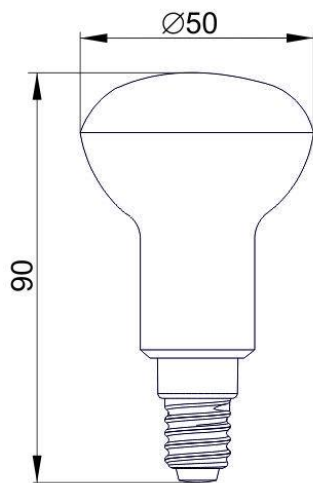
Рисунок 2 – Лампа LED-R50, 5 Вт, цоколь E14
