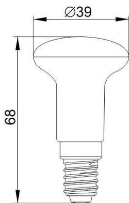
Рисунок 1 – Лампа LED-R39, 3 Вт, цоколь E14
