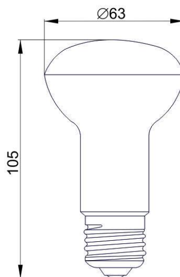
Рисунок 3 – Лампа LED-R63, 5 Вт, 8 Вт, цоколь E27
