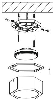
Рисунок 5 – Схема монтажа светильников типа 5204, 5304
