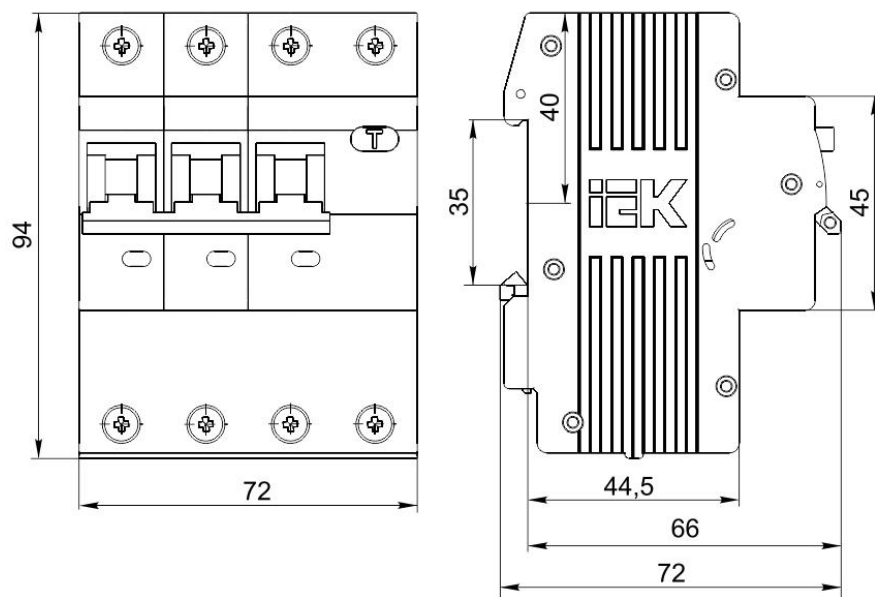
Рисунок 3 – Габаритные размеры АВДТ34
