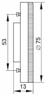
Лампа LED-T75, 4 Вт, цоколь GX53
