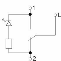
выключатель одноклавишный проходной с индикацией
