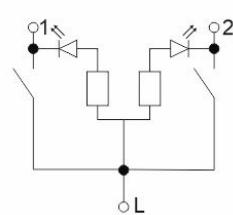
выключатель двухклавишный с индикацией
