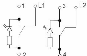
выключатель двухклавишный проходной с индикацией
