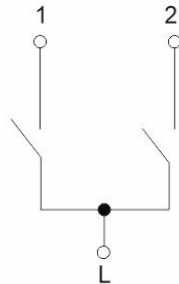
выключатель двухклавишный
