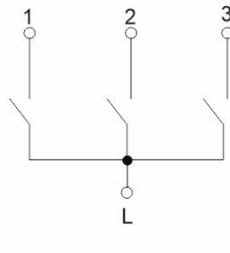
выключатель трехклавишный
