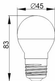
Рисунок 2 – Лампа LED-G45, 3 Вт, цоколь E27
