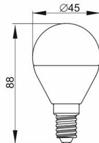
Рисунок 3 – Лампа LED-G45, 5 Вт цоколь E14
