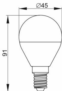
Рисунок 5 – Лампа LED-G45, 7 Вт, 9 Вт, цоколь E14
