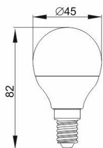
Рисунок 1 – Лампа LED-G45, 3 Вт, цоколь E14
