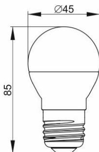
Рисунок 4 – Лампа LED-G45, 5 Вт цоколь E27
