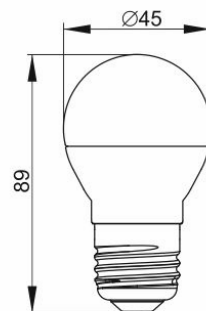
Рисунок 6 – Лампа LED-G45, 7 Вт, 9 Вт, цоколь E27
