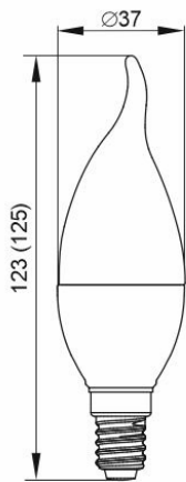
Лампа LED-СВ35, 5 Вт цоколь E14
