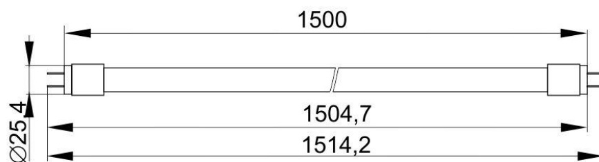
Рисунок 3 – Лампа LED-T8, 24 Вт, цоколь G13
