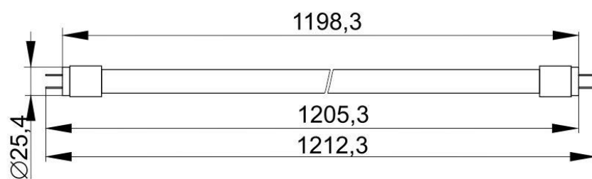
Рисунок 2 – Лампа LED-T8, 18 Вт, цоколь G13
